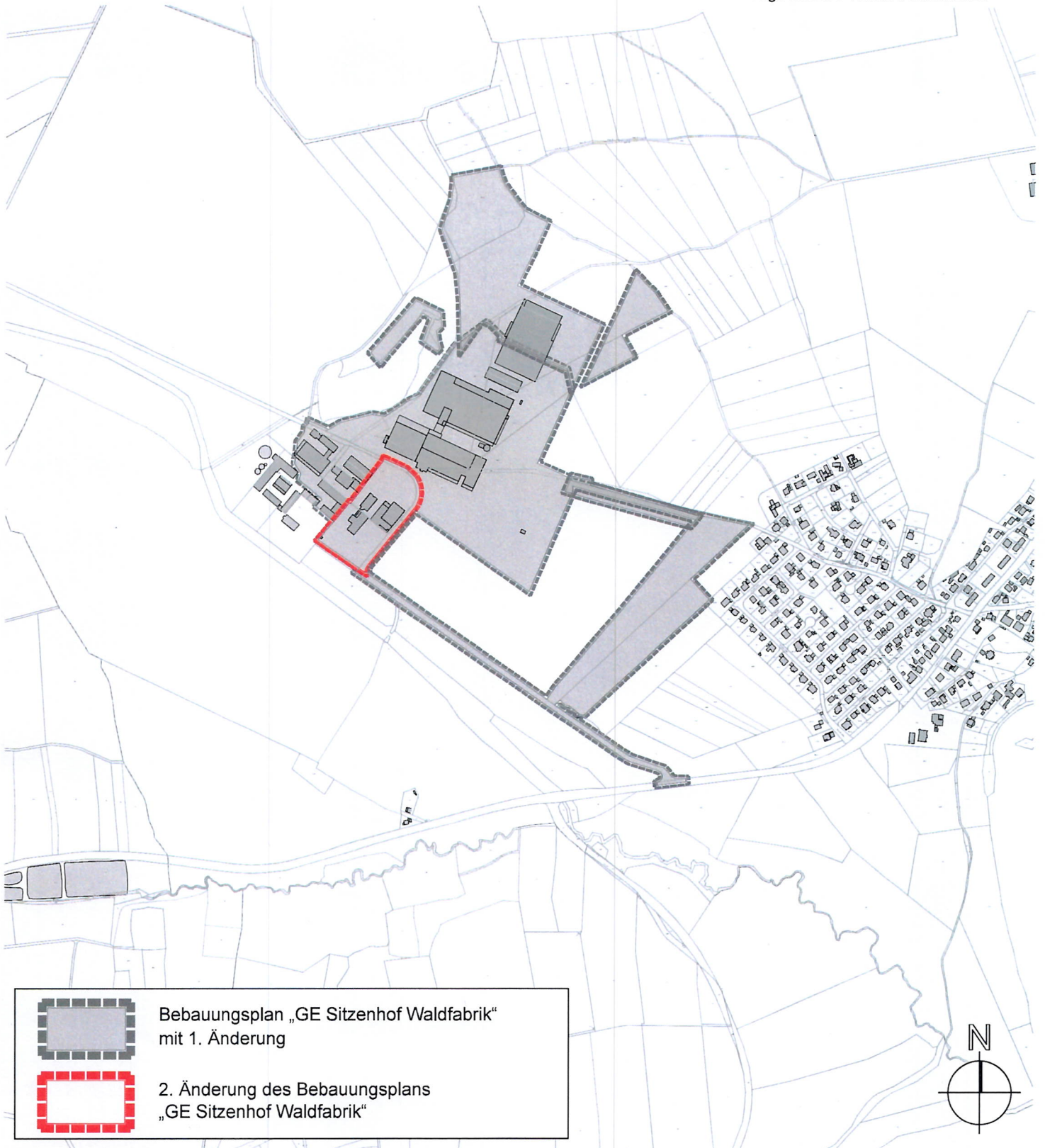
Übersichtslageplan 1:10.000
